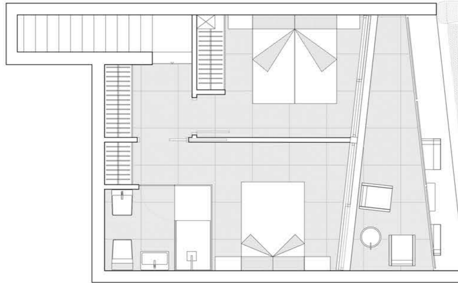
planta superior
